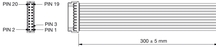
.3m 와이어를 부착한 제어 커넥터 인터페이스의 주문 키트 부품 번호 73-788-001
