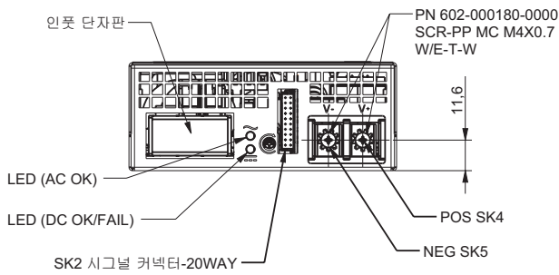
PSU 전면 모습
